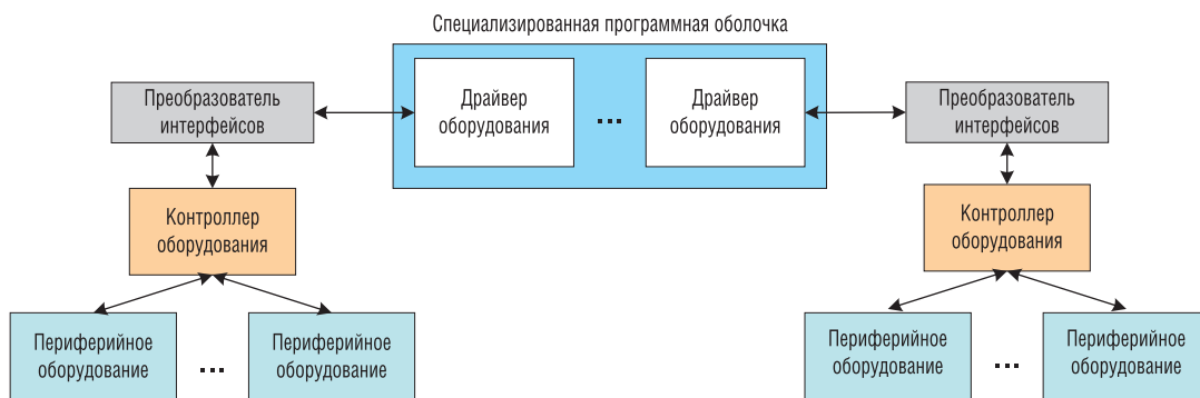
Рис. 3. Аппаратно-программная интегрированная система
