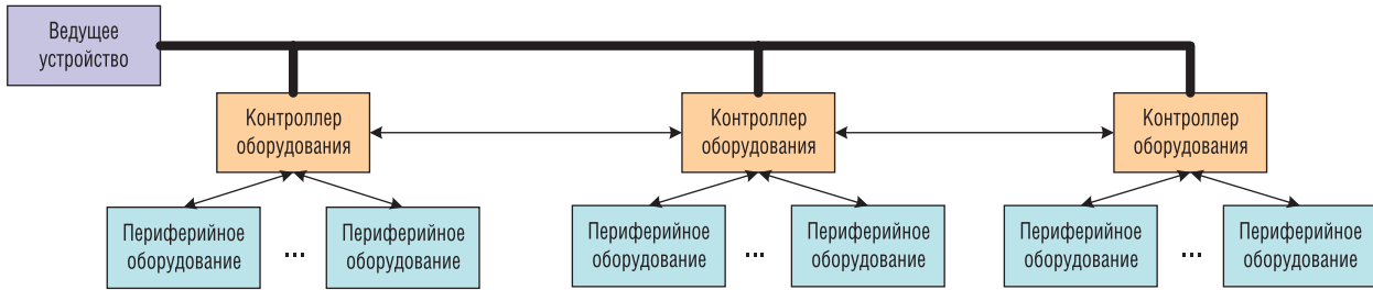
Рис. 1. Аппаратно-интегрированная система
