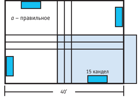
Рис. 6. Потолочная установка. Распределение в нижней полусфере
