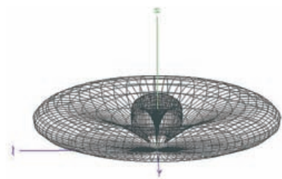
Рис. 7. Типовая диаграмма направленности коллинеарной антенны
