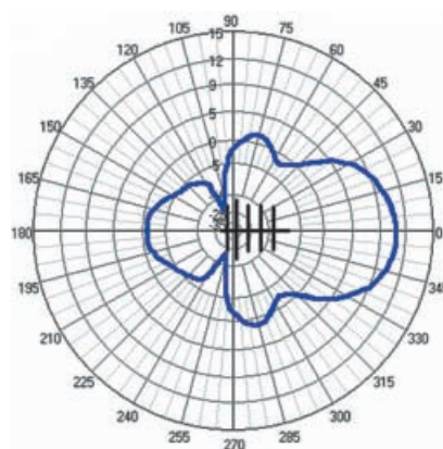
Рис. 2. Диаграмма направленности антенны «волновой канал» в горизонтальной плоскости
