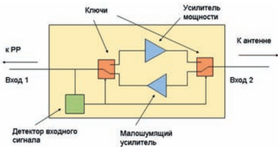
Рис. 15. Структурная схема двунаправленного усилителя радиосигнала
