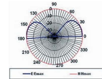
Рис. 8. Внешний вид антенны «Шайба» и ее диаграмма направленности в вертикальной и горизонтальной плоскостях
