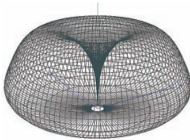
Рис. 5. Типовая диаграмма направленности антенны 5/8 λ.
