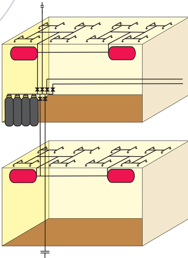
Рис. 2. Многоэтажный объект
