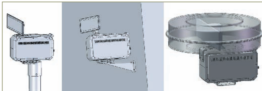
Рис. 3. Варианты установки РЛС охраны периметра и территории объектов
