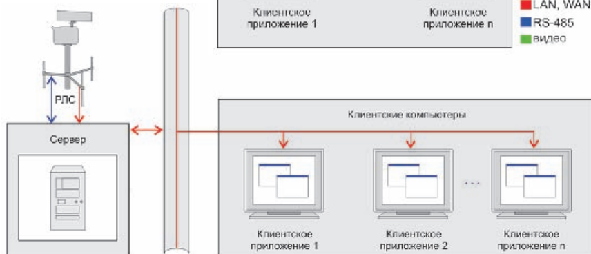
Рис. 4. Базовый вариант с сетевой архитектурой
