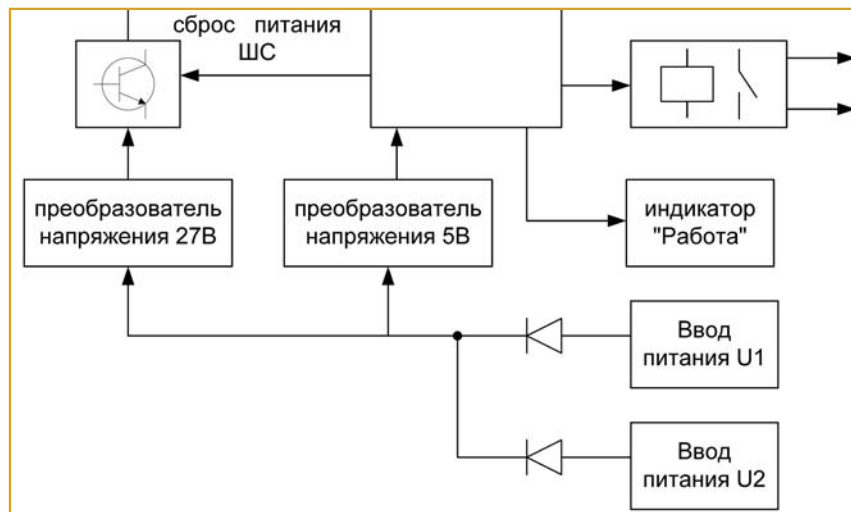
Рис. 2. Развязка двух вводов источников питания при помощи диодов
