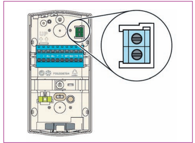
Рис. 8. Дополнительные клеммы
