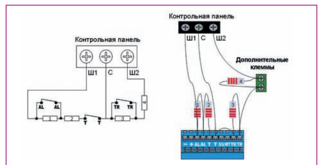
Рис. 9. Подключение шлейфов с использованием дополнительных клемм
