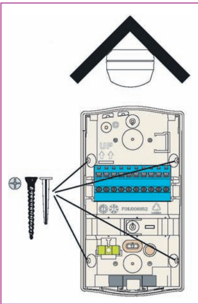
Рис. 3. Боковые ребра для монтажа извещателя в углу
