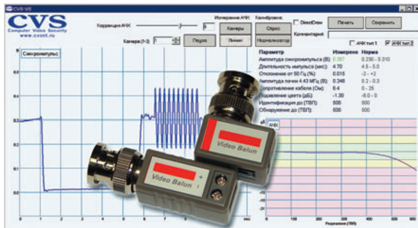
Рис. 1. Характеристики пассивных приемопередатчиков
