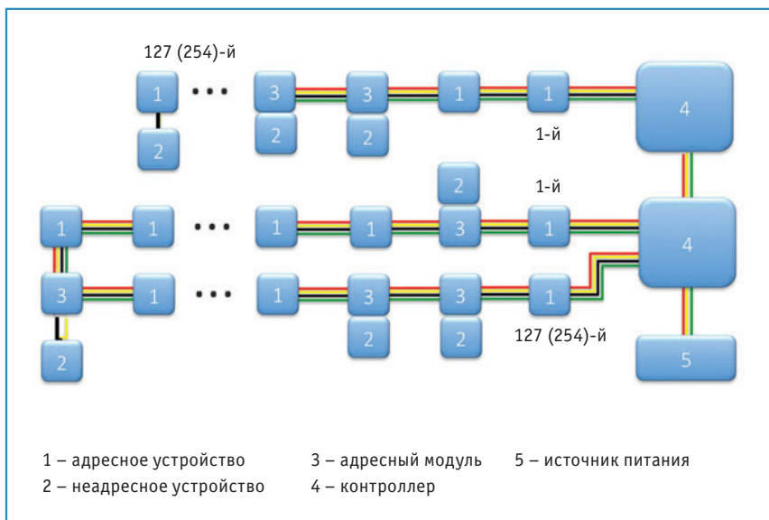
Рис. 5. Сеть с 2 изоляторами в каждом адресном модуле (технология LSN Bosch)
