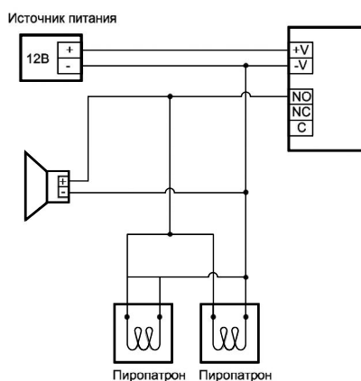
Рис. 1. Схема подключения КПО-1
